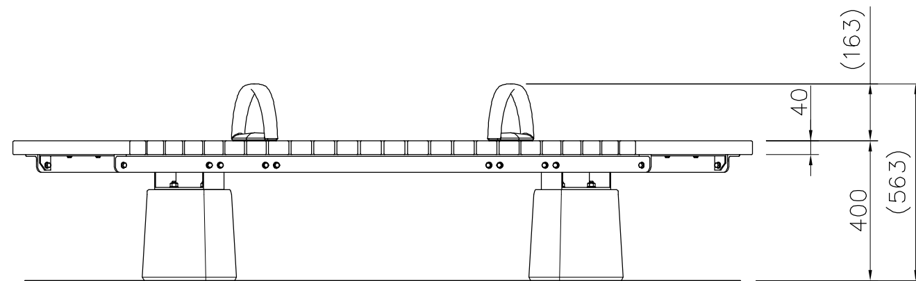
外観図 S=1/15
