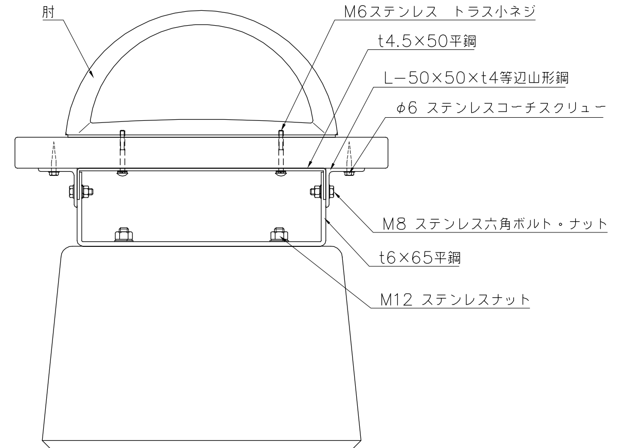
詳細図 S=1/5
