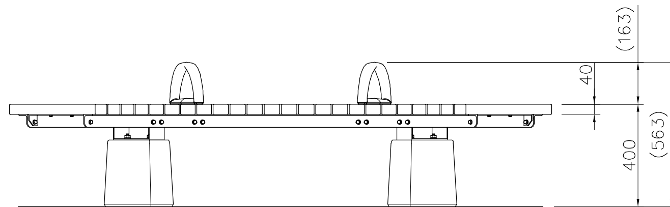
外観図 S=1/15
