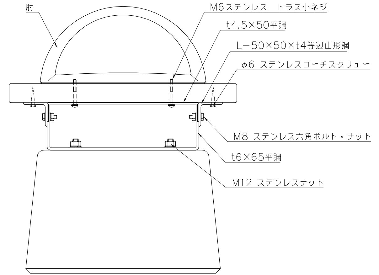
詳細図 S=1/5
