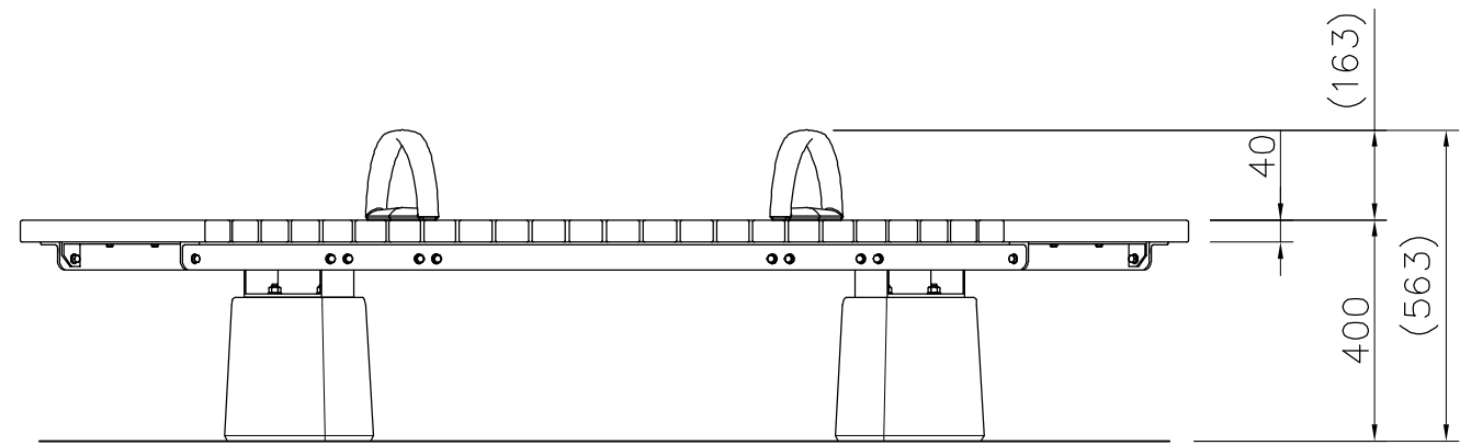
外観図 S=1/15
