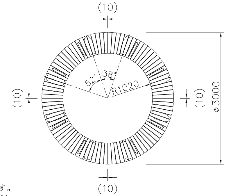
4基配置図 S=1/50
