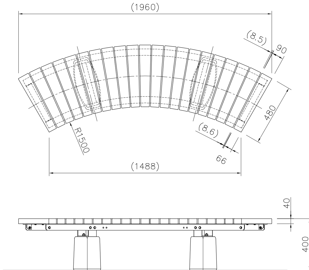
外観図 S=1/15
