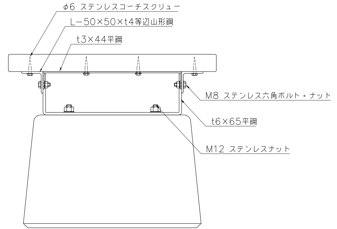
詳細図 S=1/5
