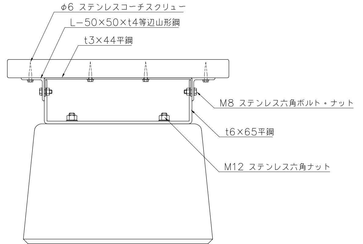
詳細図 S=1/5
