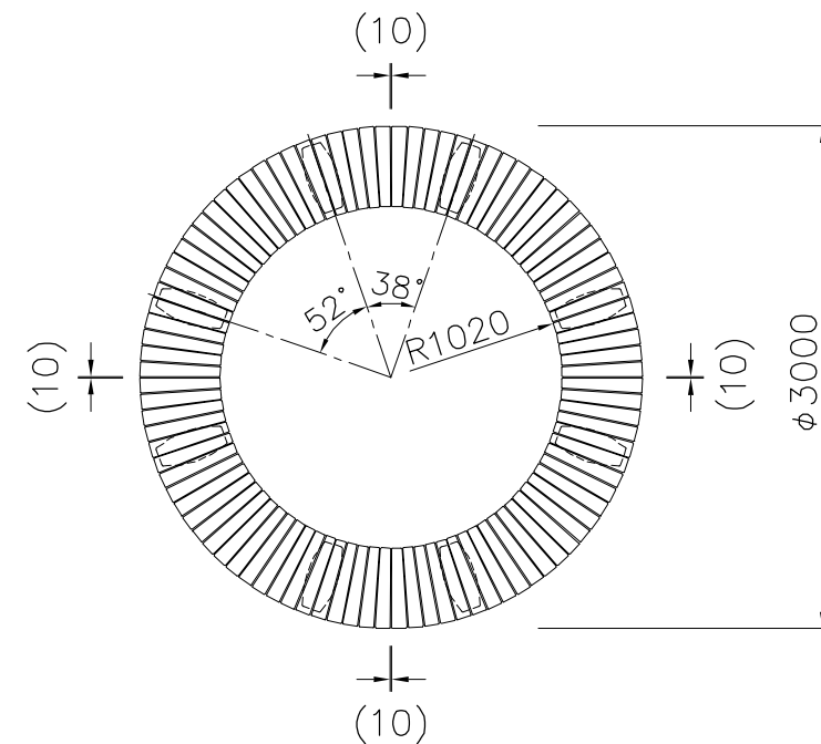
4基配置図 S=1/50
