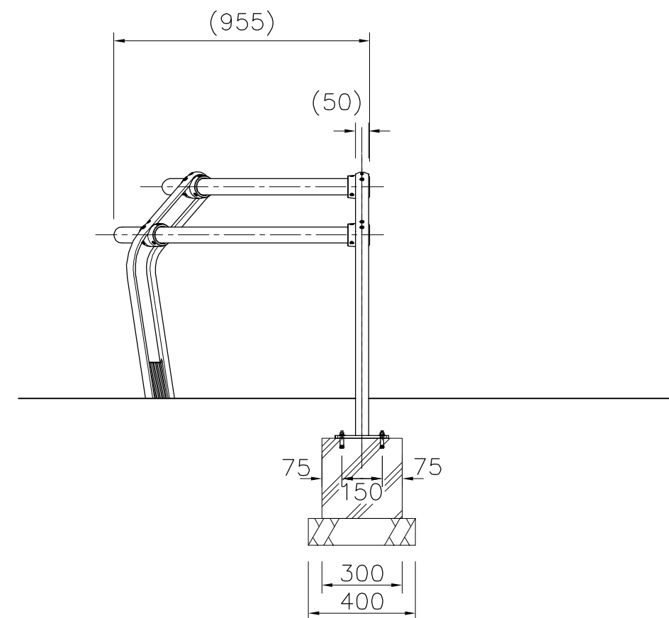
外観図 S=1/20
