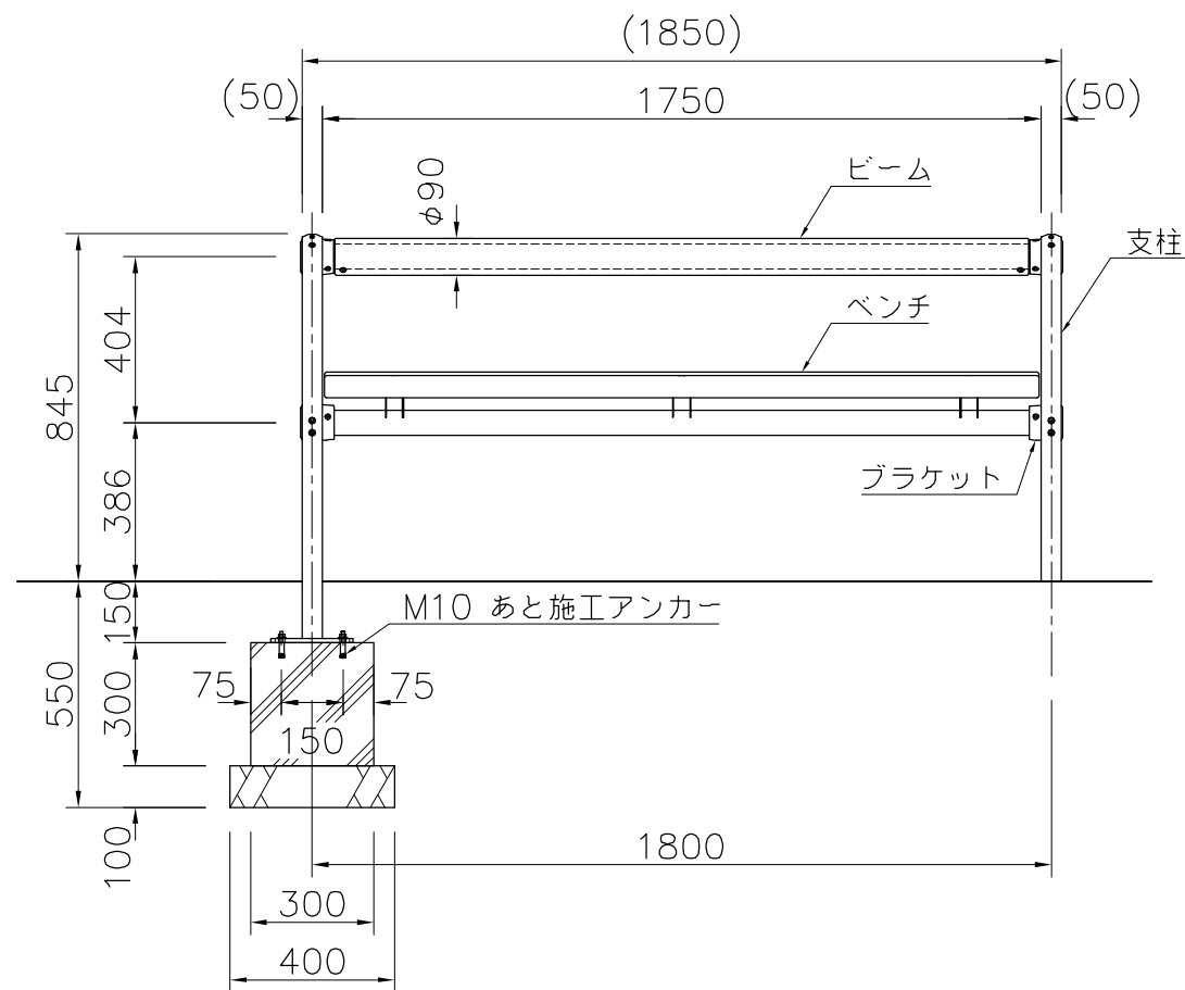
外観図 S=1/20
