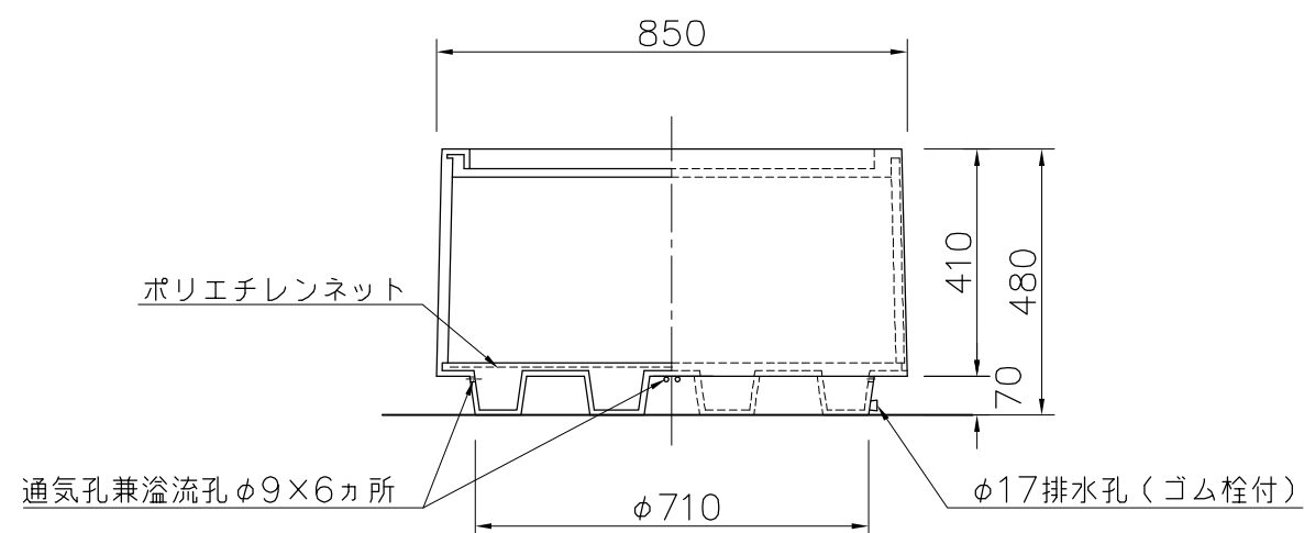
外観図 S=1/15
