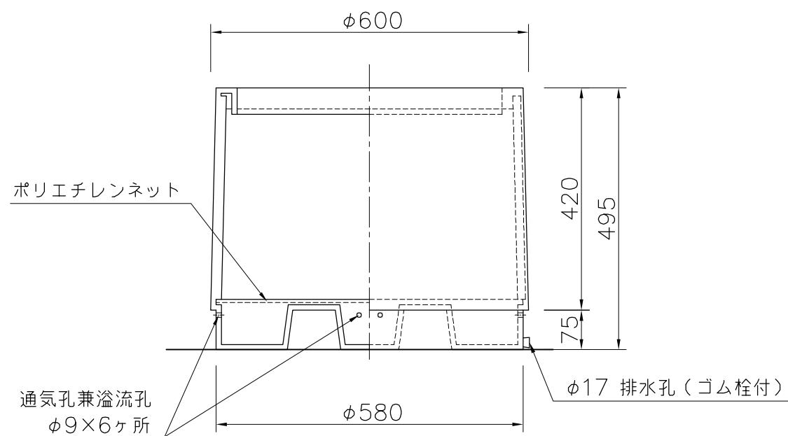
外観図 S=1/10
