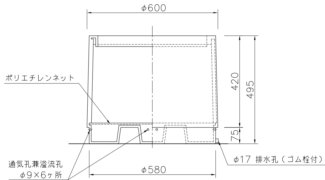
外観図 S=1/10
