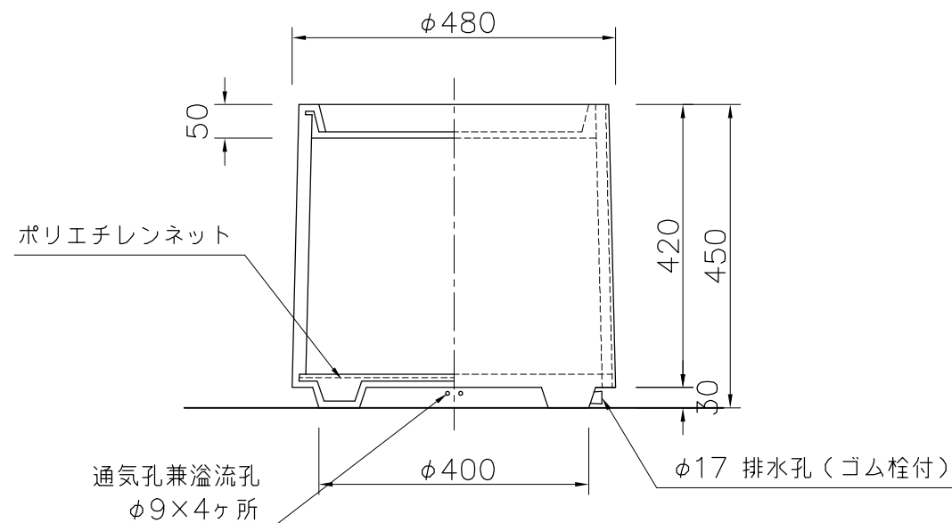
外観図 S=1/10
