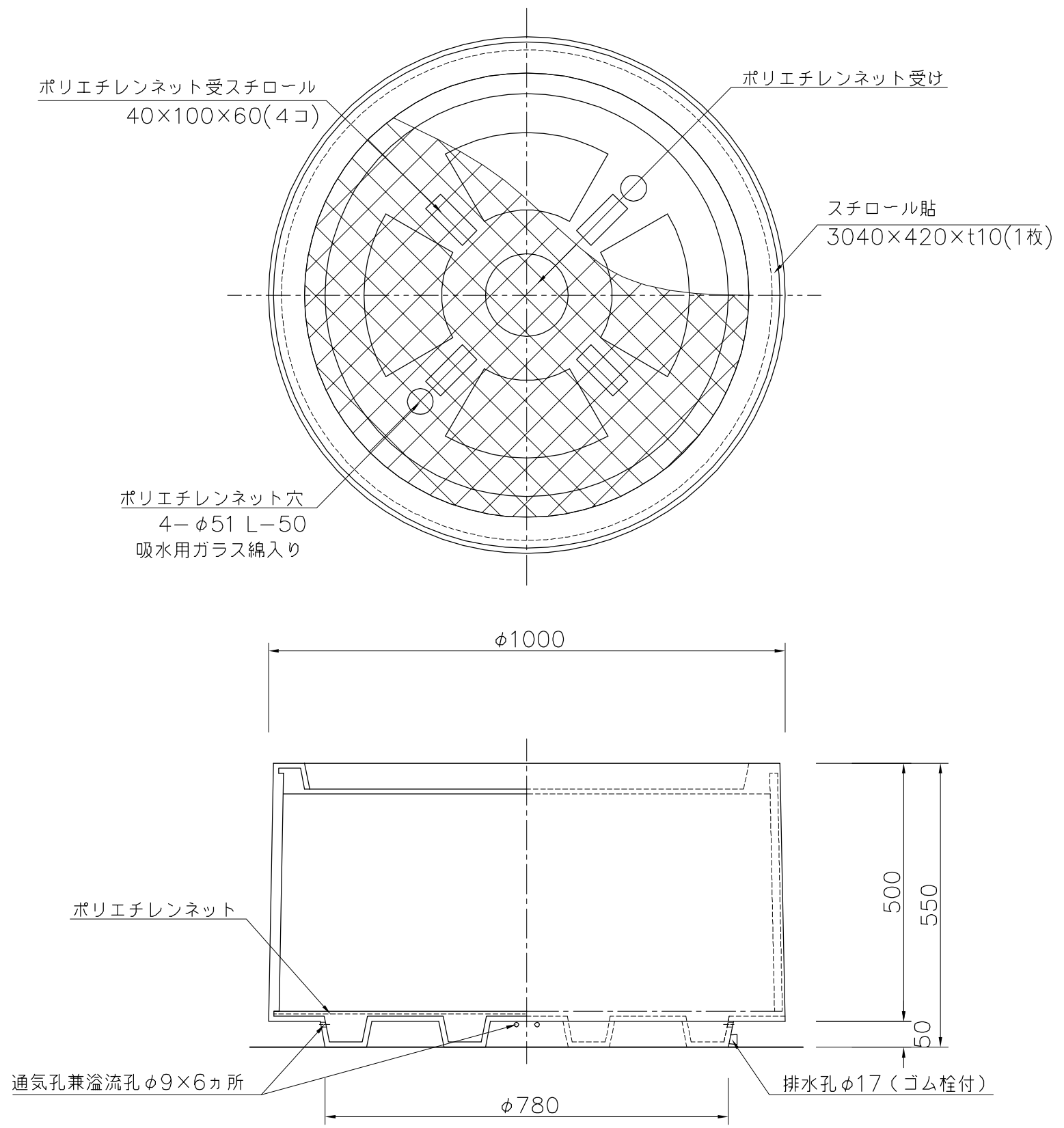
外観図 S=1/10
