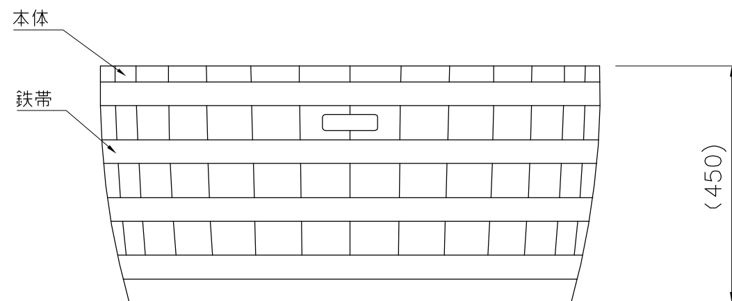
外観図 S=1/10
