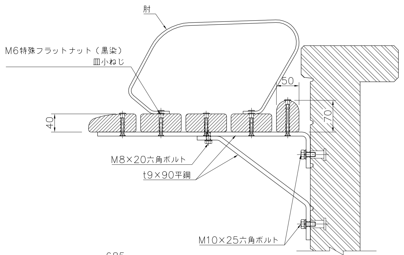
詳細図 S=1/5
