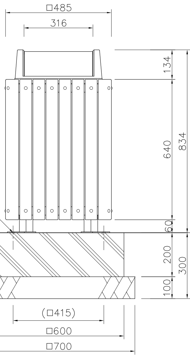
外観図
