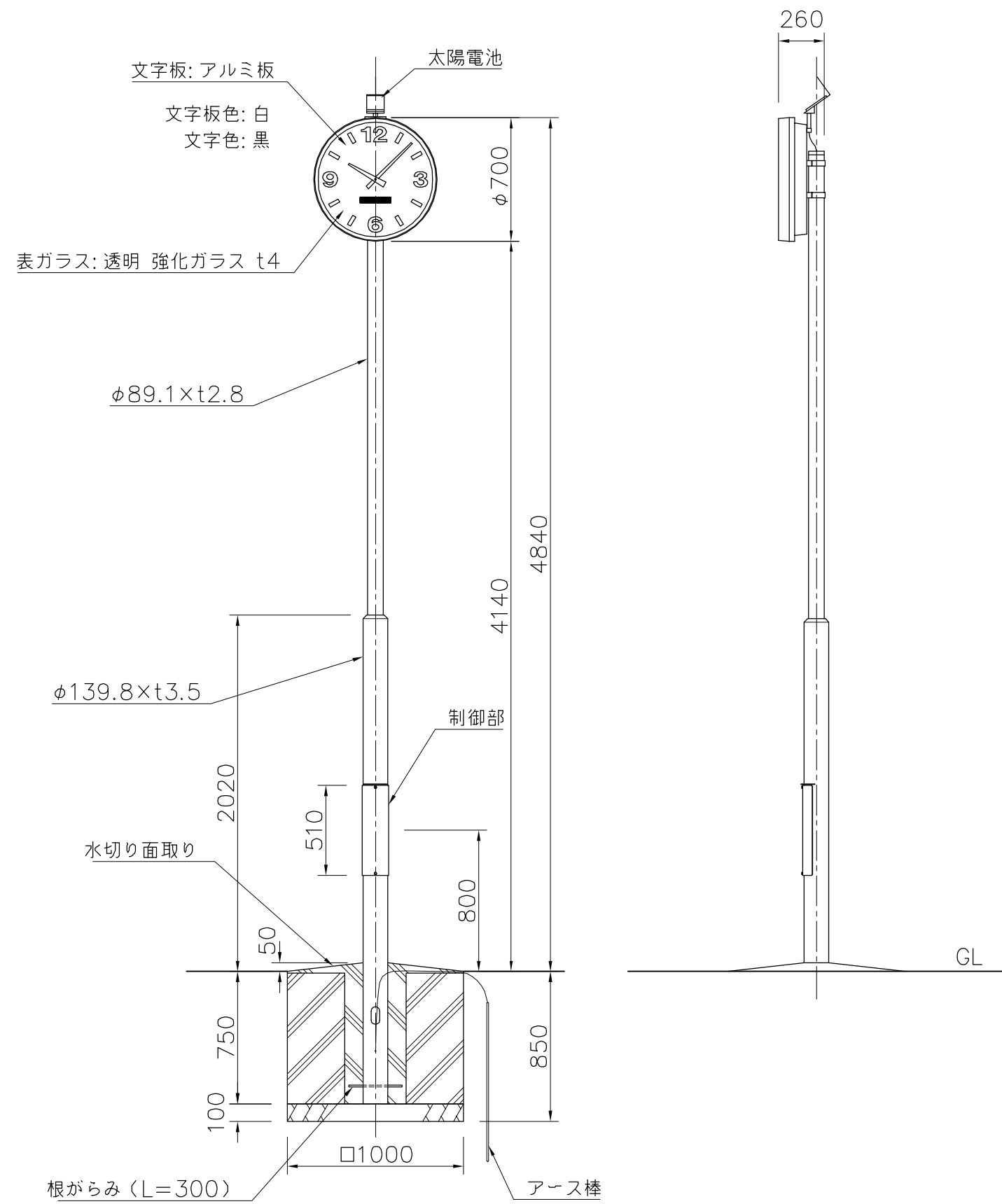
外観図 S=1/30
