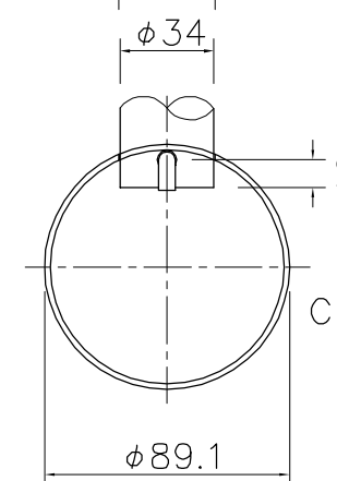
詳細図 S=1/3
