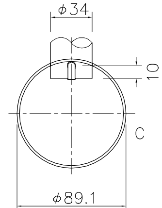
詳細図 S=1/3
