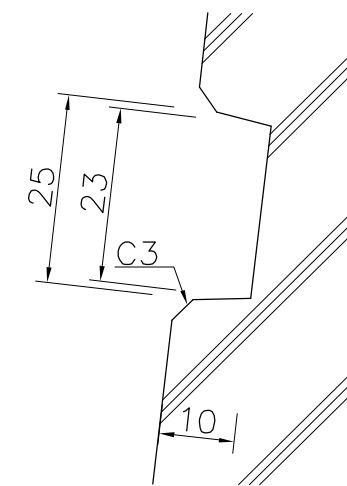
A部詳細図 S=1/1
