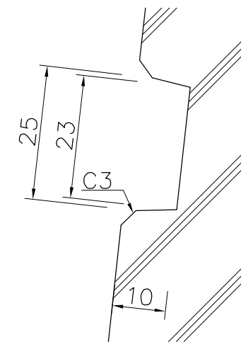
A部詳細図 S = 1 : 1
