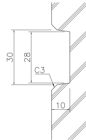
A部詳細図 S=1/1
