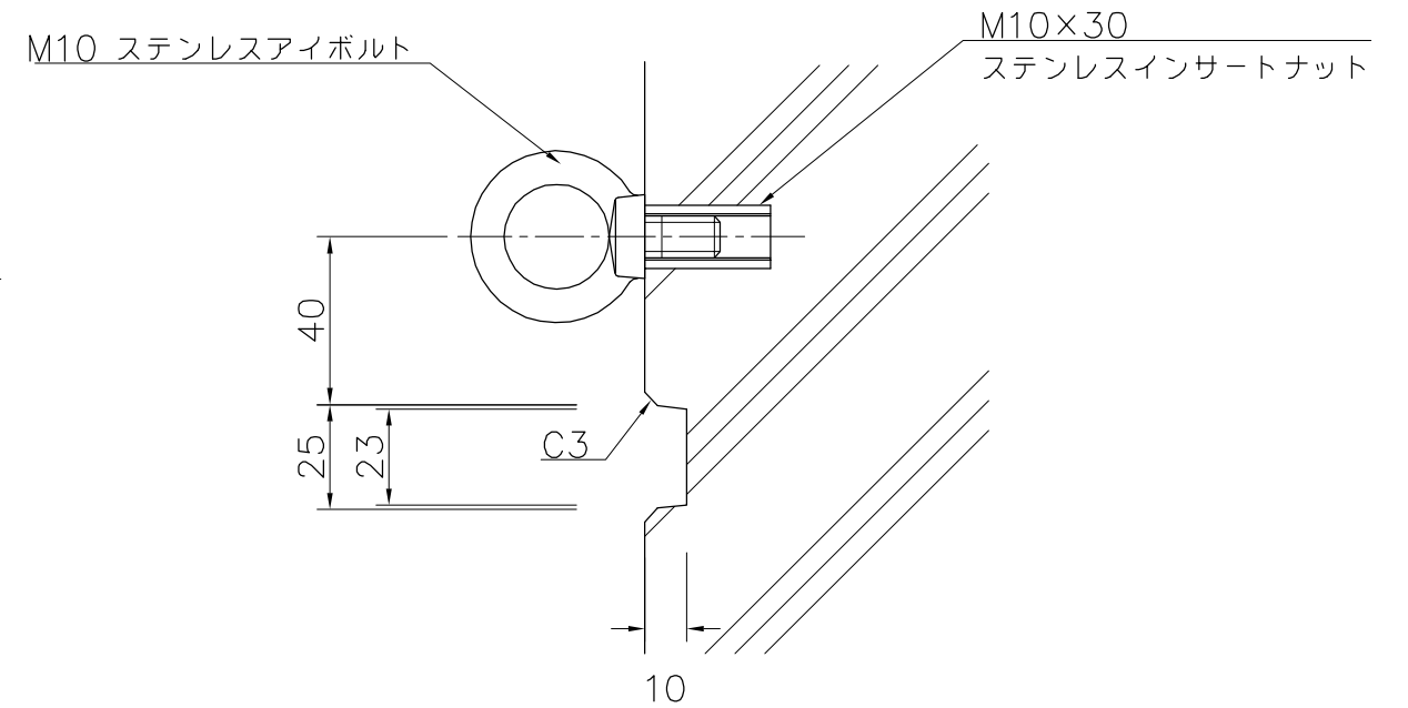
A部断面詳細図 S=1/2
