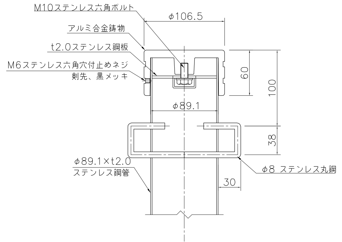
詳細図 S=1/3
