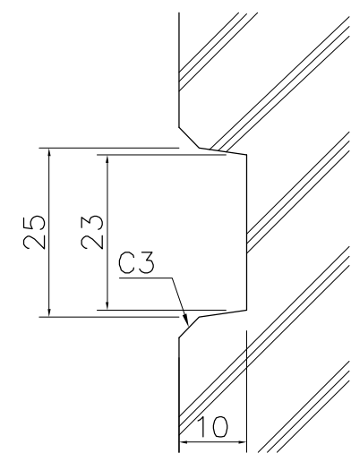
A部断面詳細図 S=1/1
