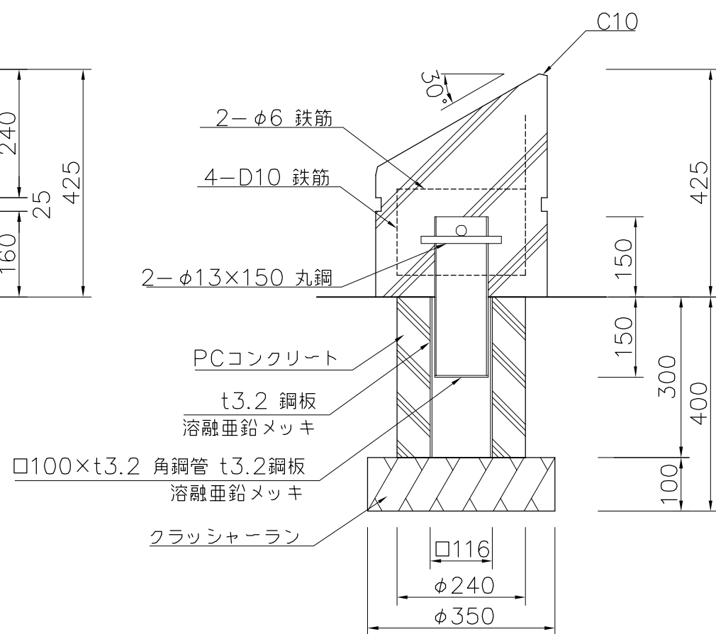
外観図 S=1/10
