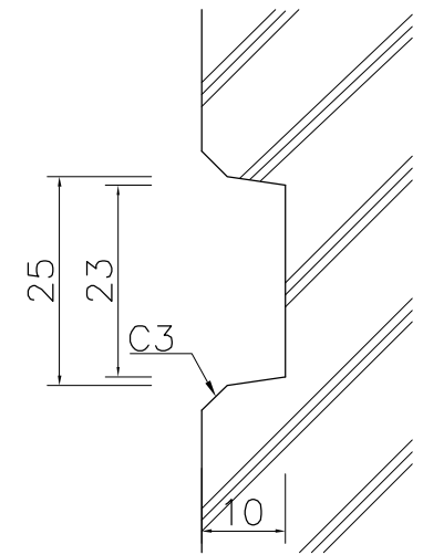
A部断面詳細図 S=1/1
