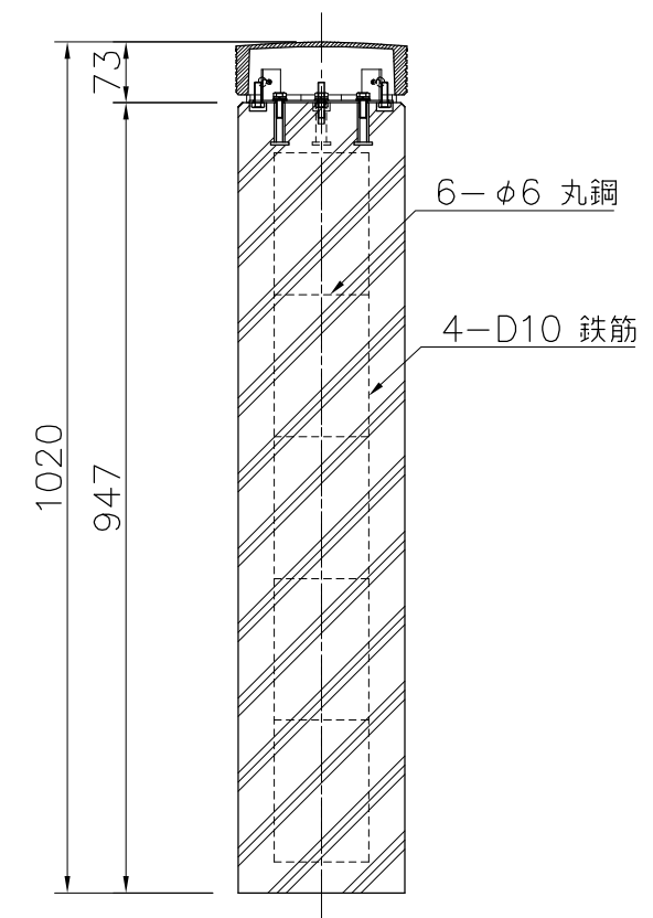
断面図 S=1/10
