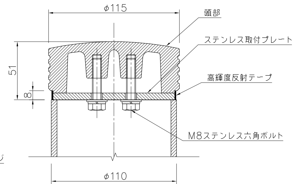
頭部取付詳細 S=1/2
