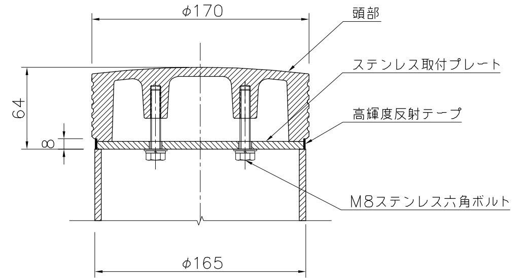
頭部取付詳細 S=1/3
