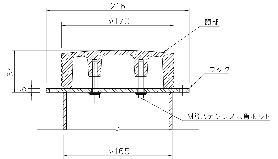
頭部取付詳細 S=1/3
