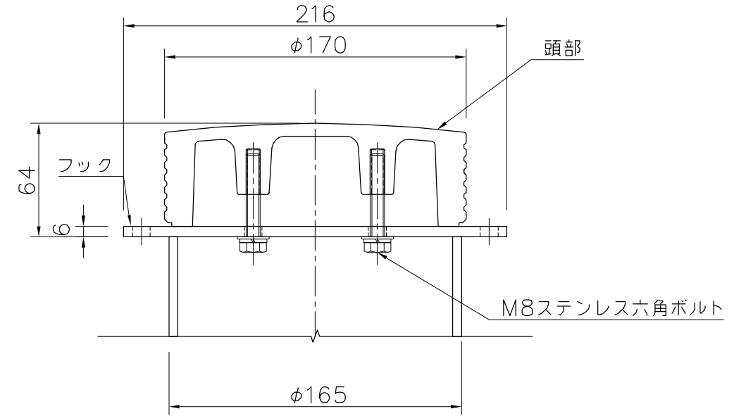
頭部取付詳細 S=1/3
