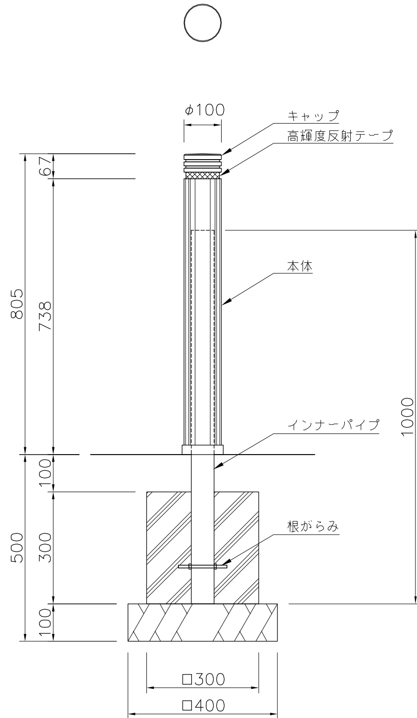
外観図 S=1/10
