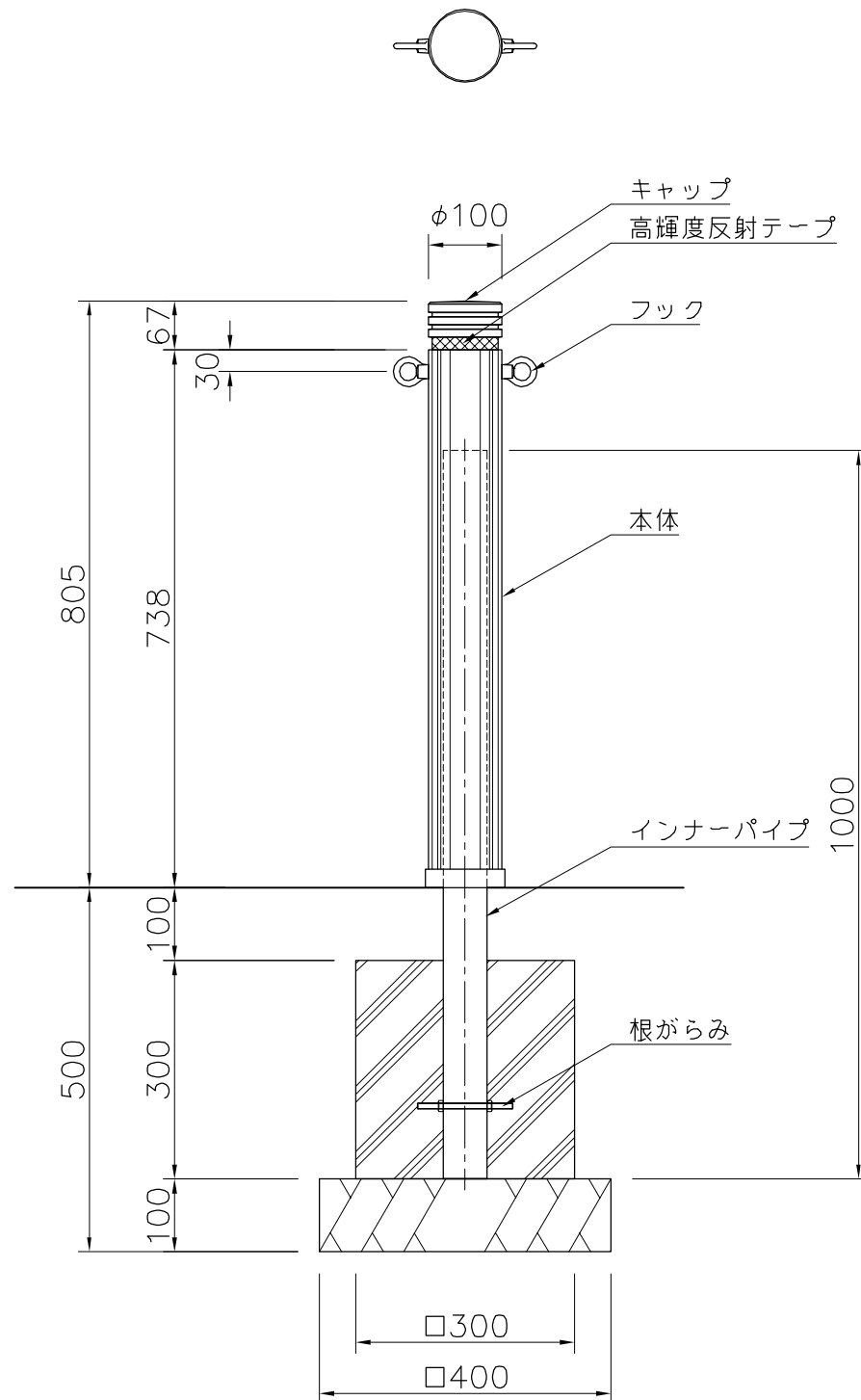
外観図 S=1/10
