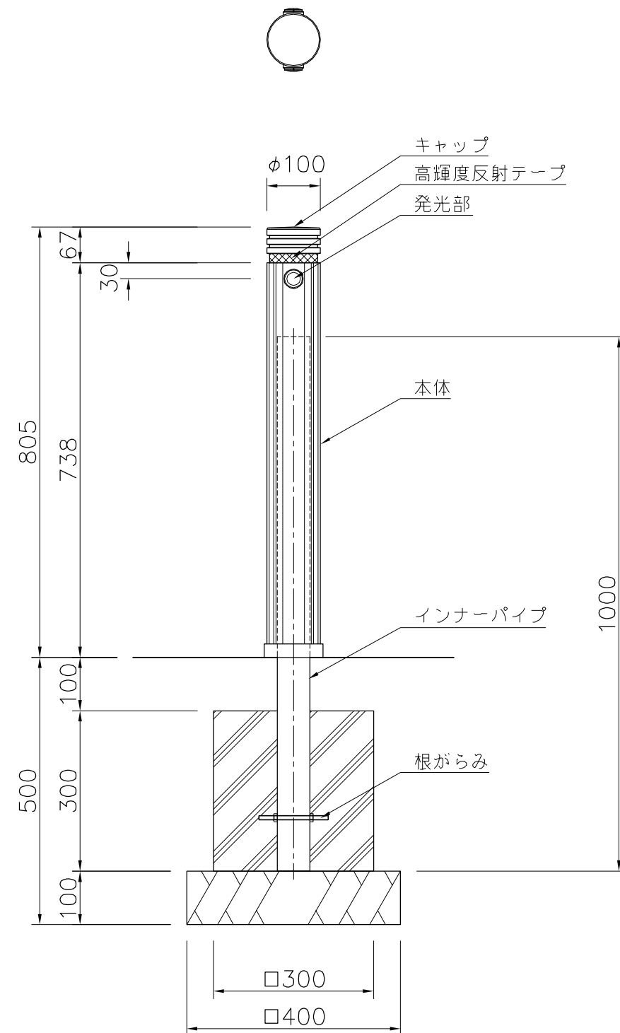
外観図 S=1/10
