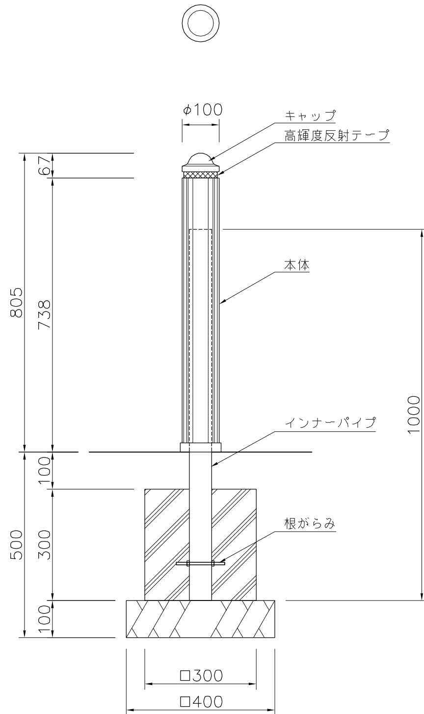
外観図 S=1/10
