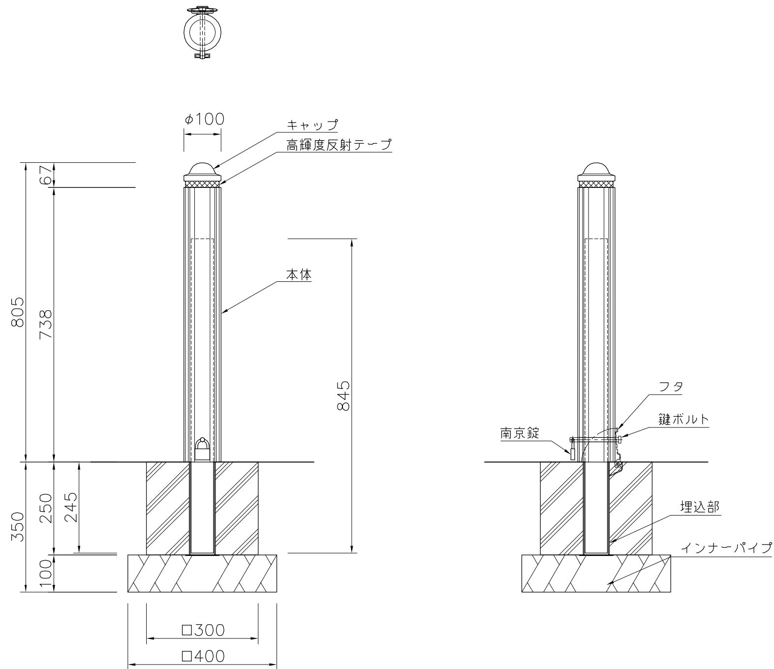
外観図 S=1/10
