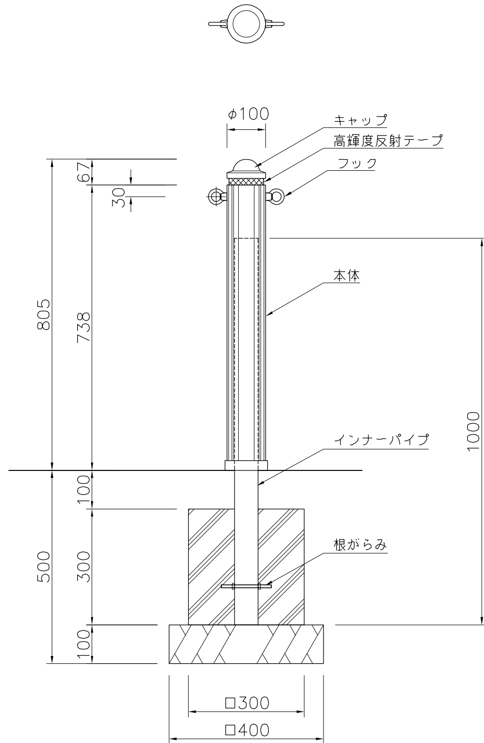
外観図 S=1/10
