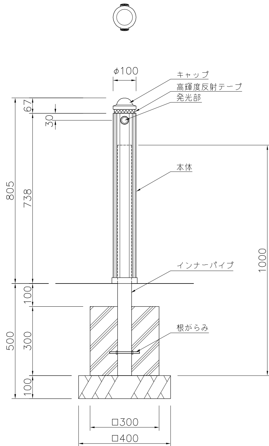
外観図 S=1/10
