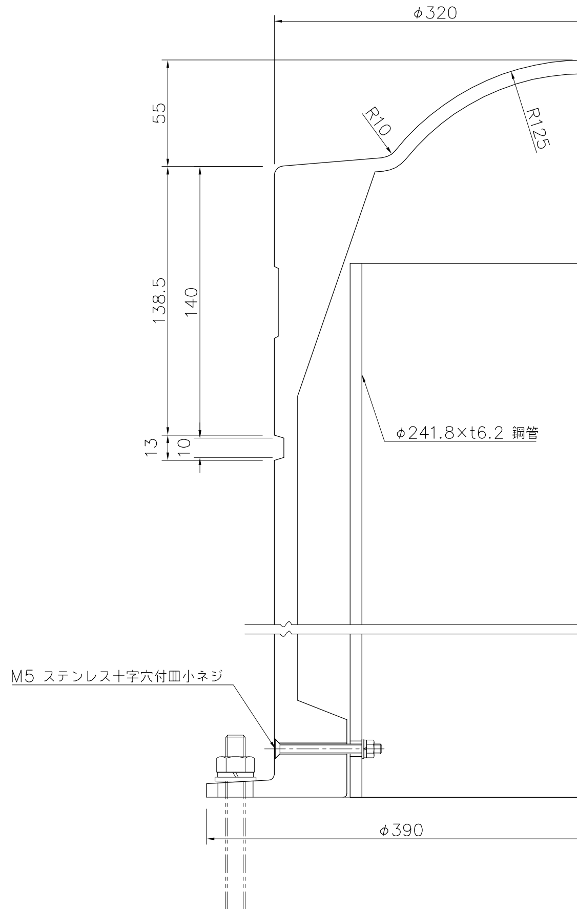
詳細図 S=1/2
