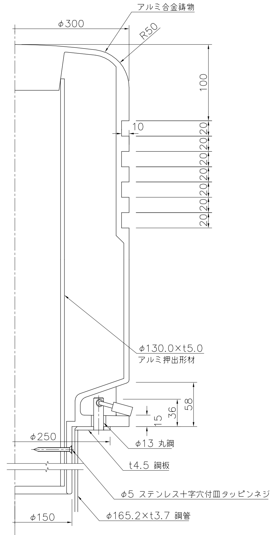
詳細図 S=1/3
