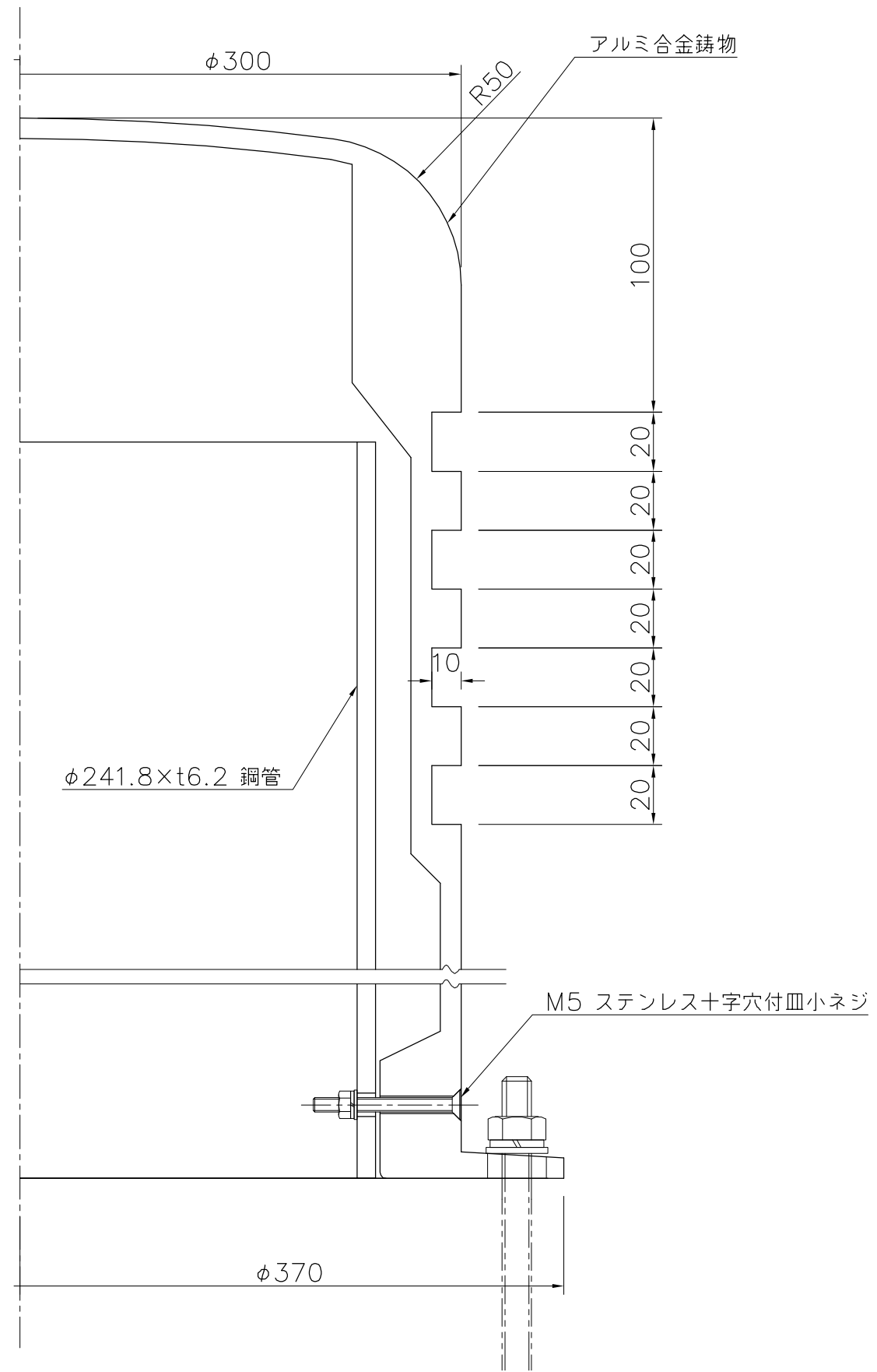
詳細図 S=1/2
