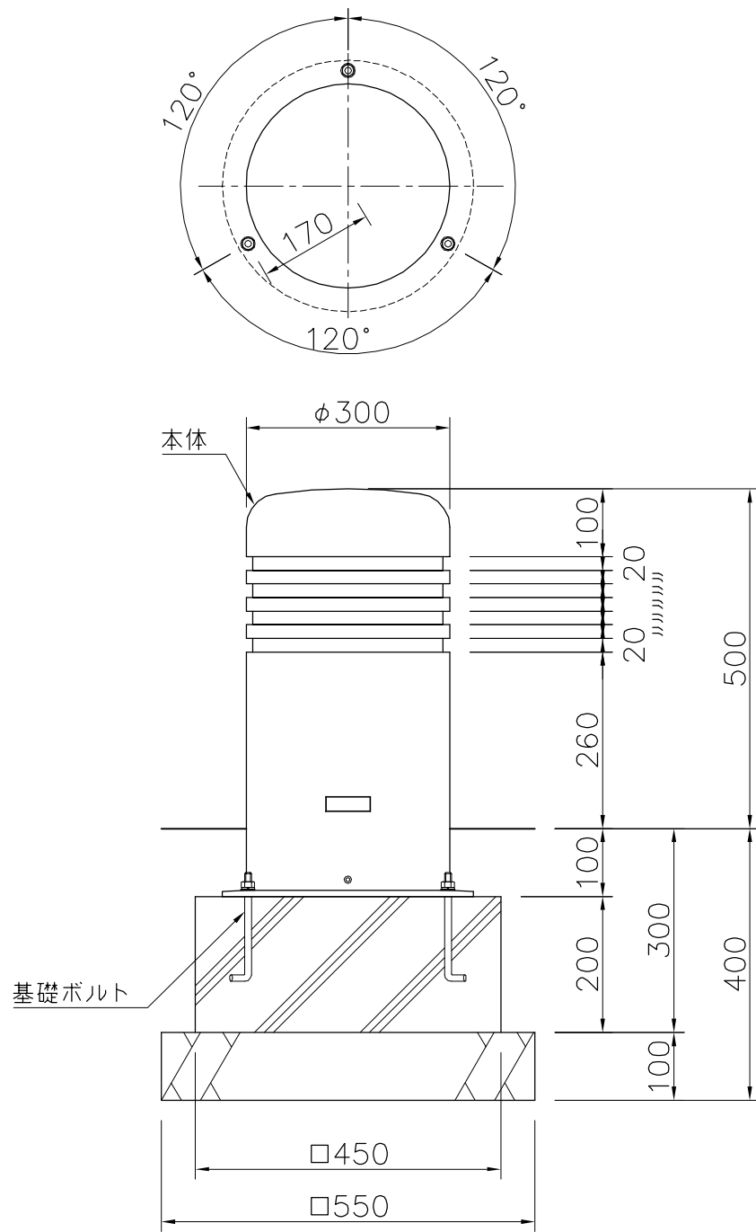
詳細図 S=1/2
