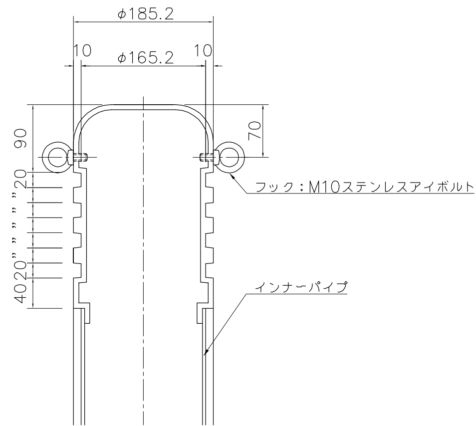
詳細図 S=1/5
