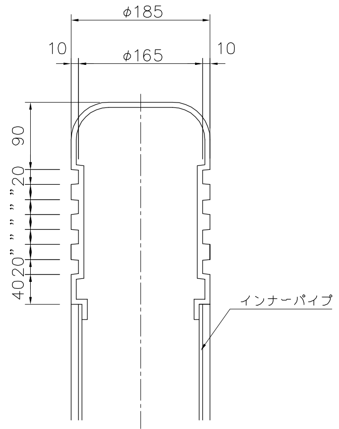
詳細図 S=1/5
