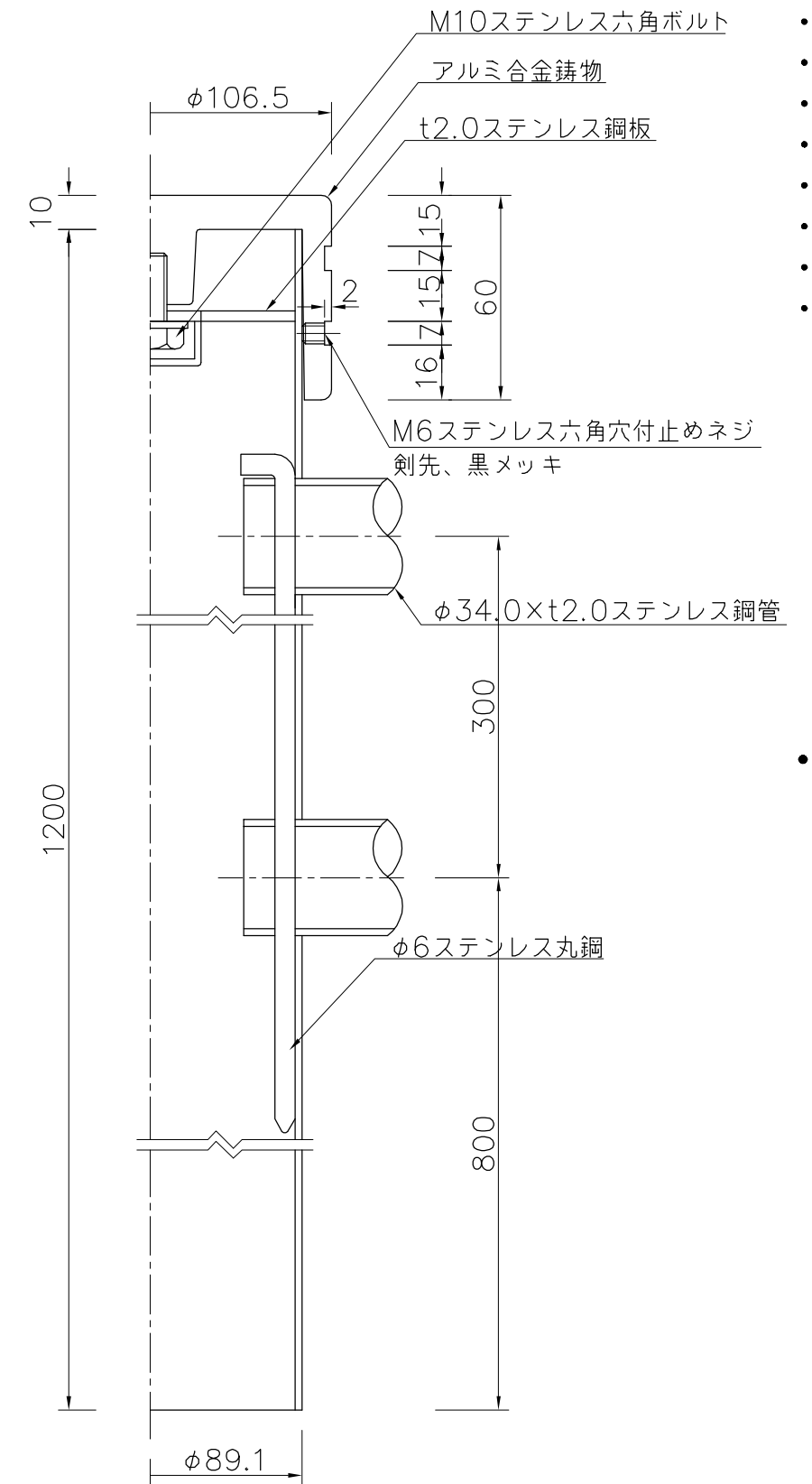
支柱断面詳細図 S = 1 : 2
