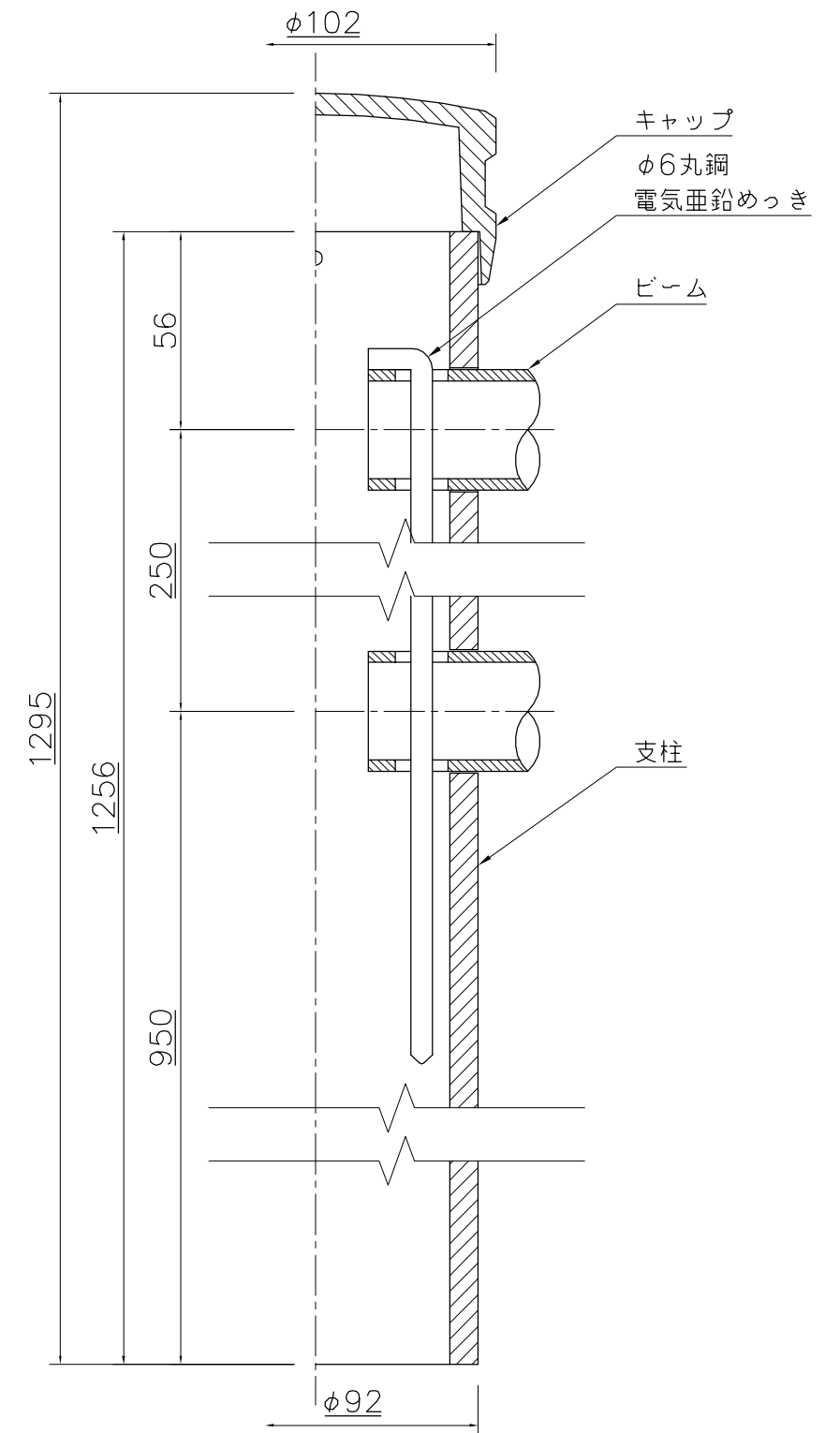
支柱断面詳細図 S=1/2
