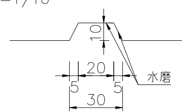
D部詳細図 S=1/2
