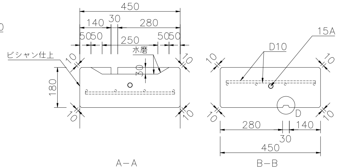
断面図 S=1/10
