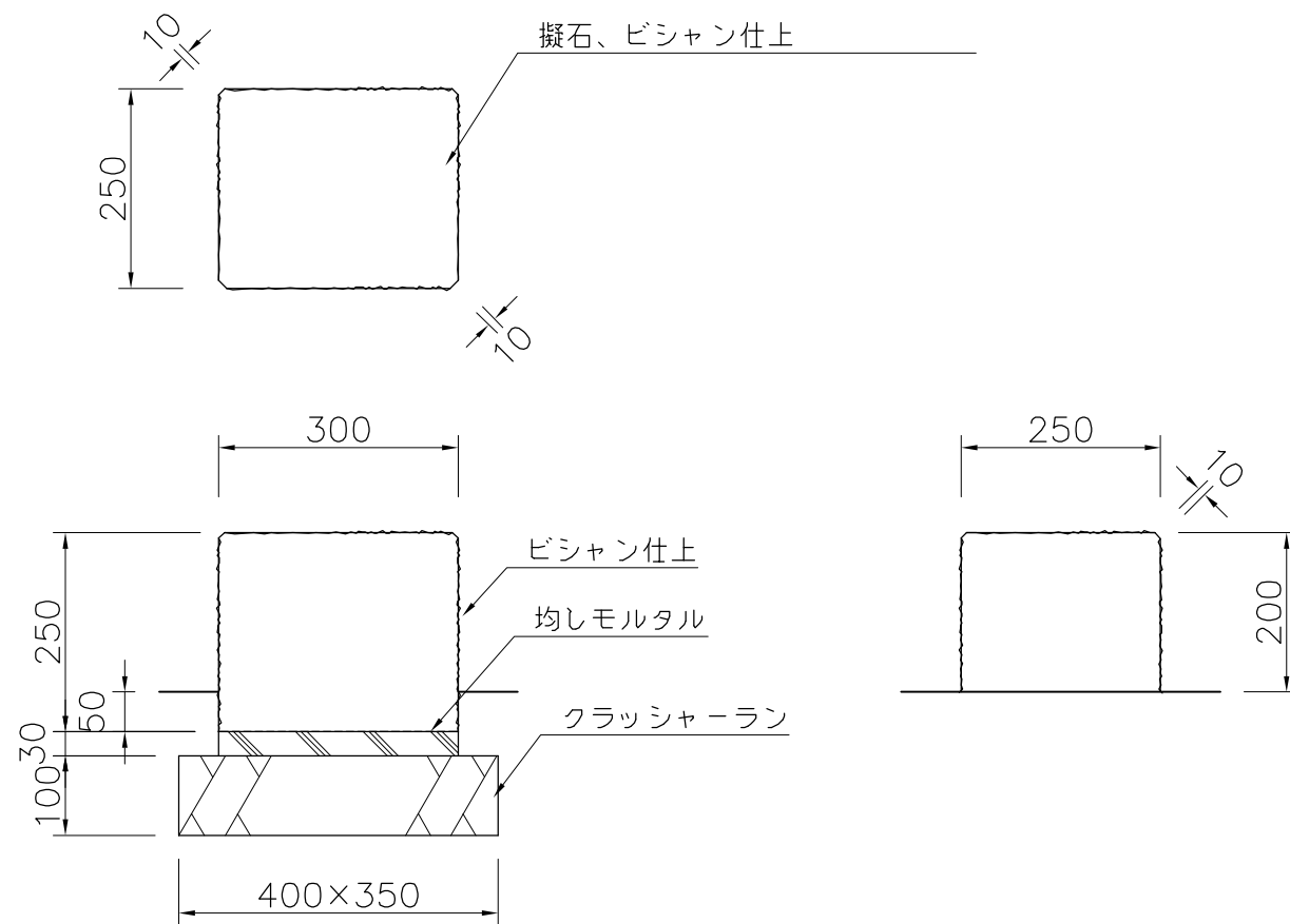
外観図 S=1/10
