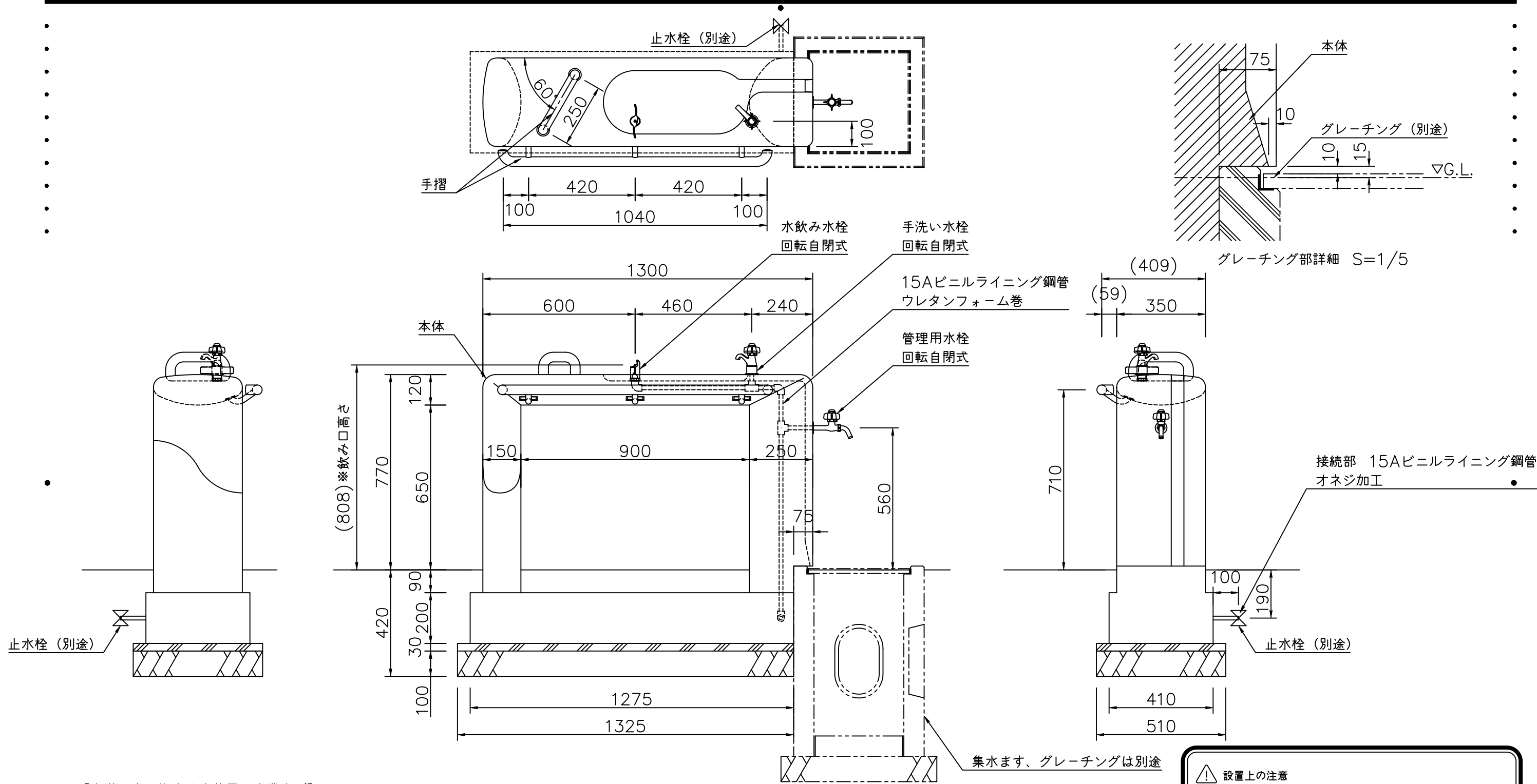
外観図 S=1/15
