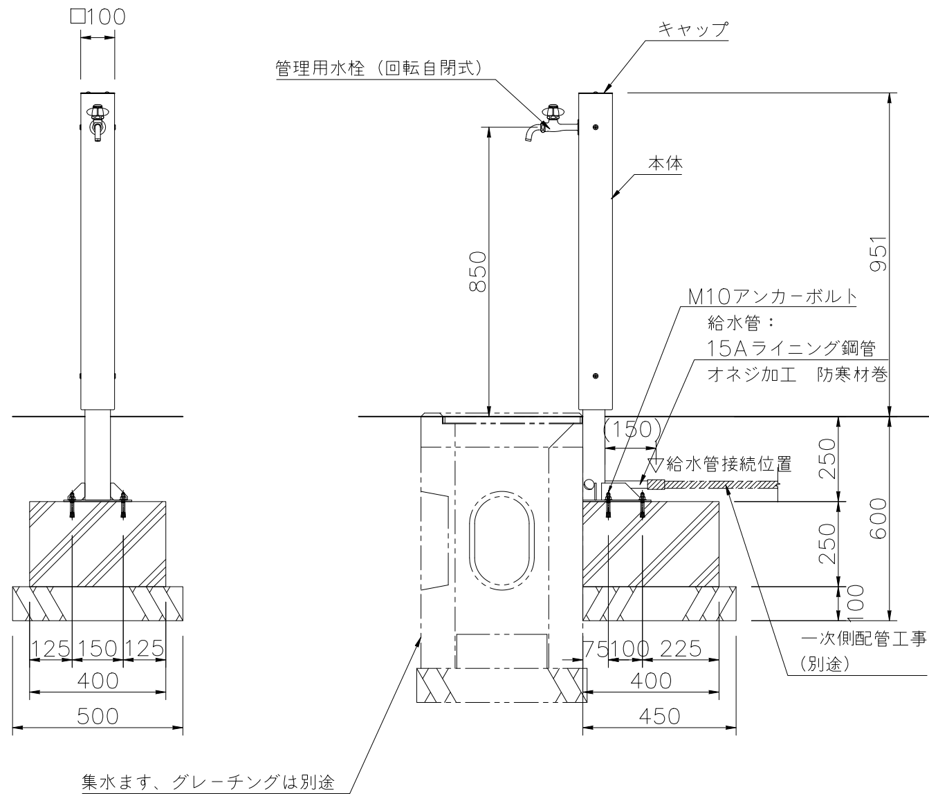
外観図 S=1/15
